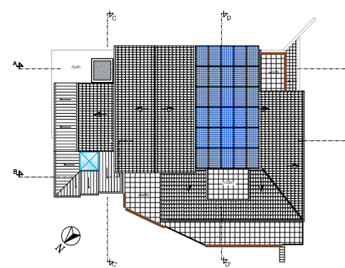
PIANTA COPERTURA
